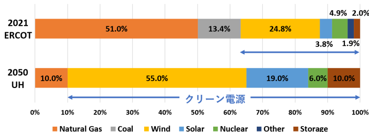
(図2) Generation Capacity in Texas (ERCOTおよびUH Center of Houston's Futureのデータから作成)
